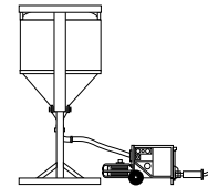
piccolo Silo mit Übergabeschlauch zur speedy P15V
